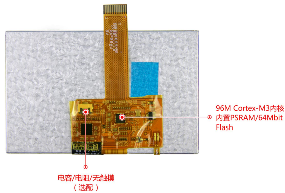
图 1-4 硬件配置图
