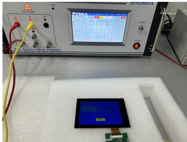
图 7-4 群脉冲测试图
